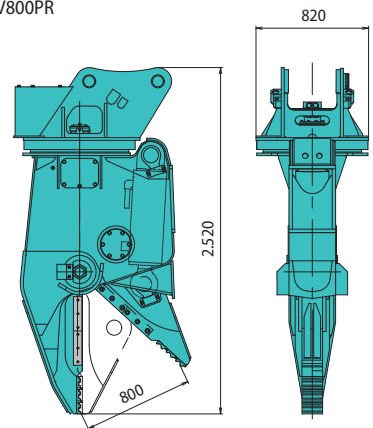
Fahrzeug-Demontagezange KV800PR
