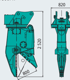
Pince de démantèlement lourd KV800PR
