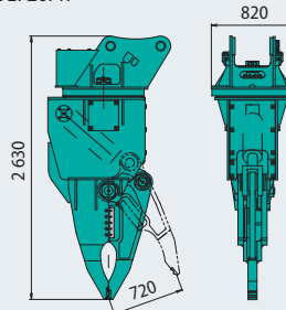
Pince de démantèlement multiple KVE720PR
