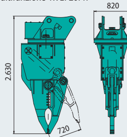
Cesoia per demolizione multifunzione KVE720PR Unità: mm
