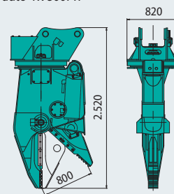
Cesoia per demolizione di auto KV800PR Unità: mm
