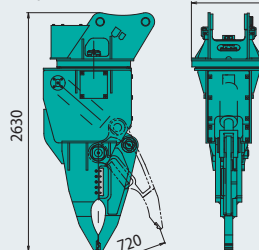
Pinza para multidesmantamiento KVE720PR Unidad: mm
