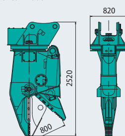
Pinza para desguace de coches KV800PR Unidad: mm
