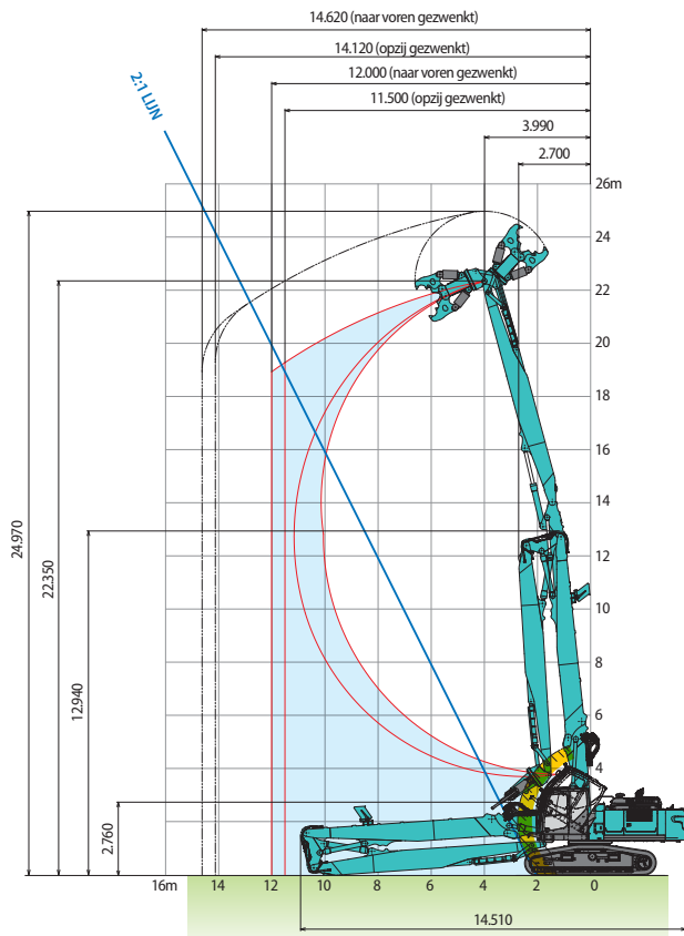
SK400D LC Graafarm van 8,7 m Max. gewicht uitrustingsstuk = 2.600 kg
