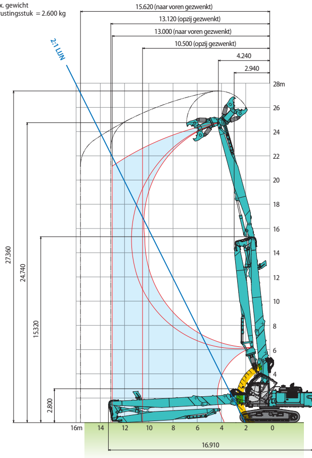
SK400D LC Graafarm van 8,7 m Max. gewicht uitrustingsstuk = 2.600 kg
